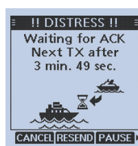
Écran ASN
