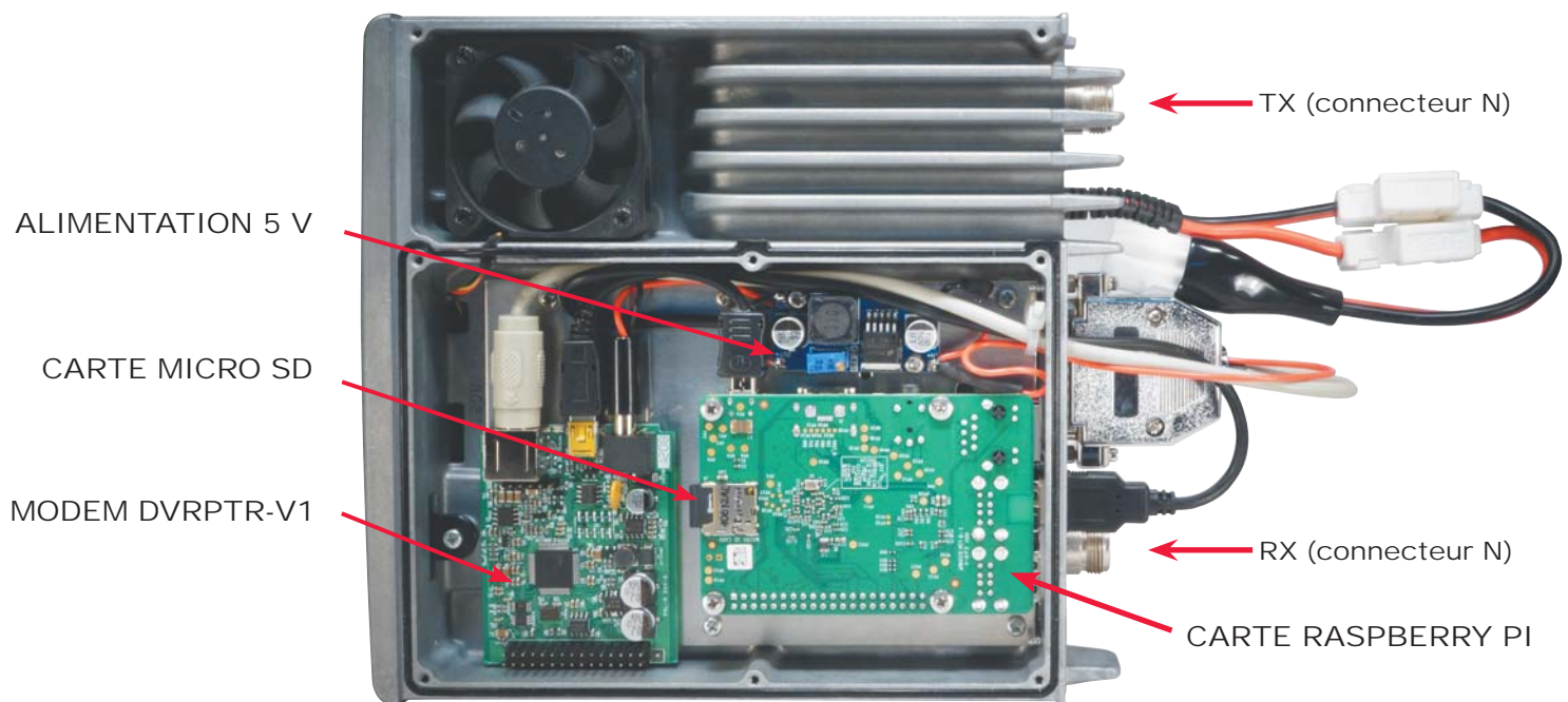
Vue de dessus Photo capot ouvert avec exemple de montage du kit D-STAR
